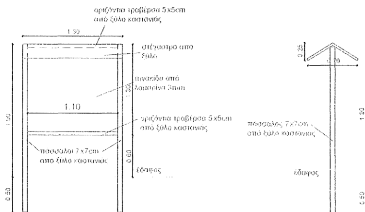
ΕΙΚΟΝΑ 1. ΟΨΗ-ΤΟΜΗ ΠΙΝΑΚΙΔΑΣ ΕΡΜΗΝΕΙΑΣ ΠΕΡΙΒΑΛΛΟΝΤΟΣ
